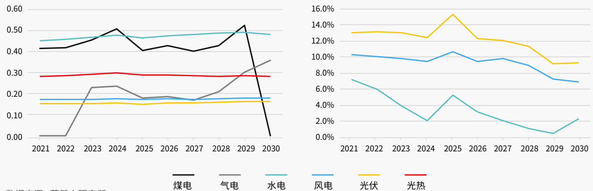
图表 17 基准政策情景各机组类型容量因子(左)和可再生能源弃电率(右)
