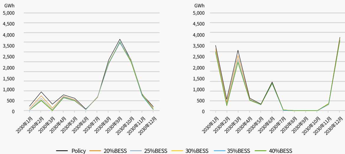
图表 21 不同储能配比情景2030年月度弃风弃光总量(左)和外购量(右)
