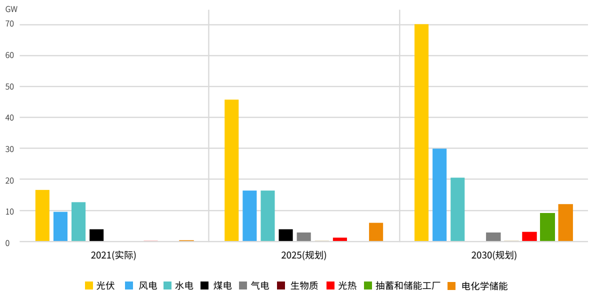
图表 2 青海2021现状以及2025/2030电源装机目标
