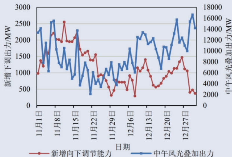
图表40 山西现货申报新增向下调能力与中午风光叠加对比
