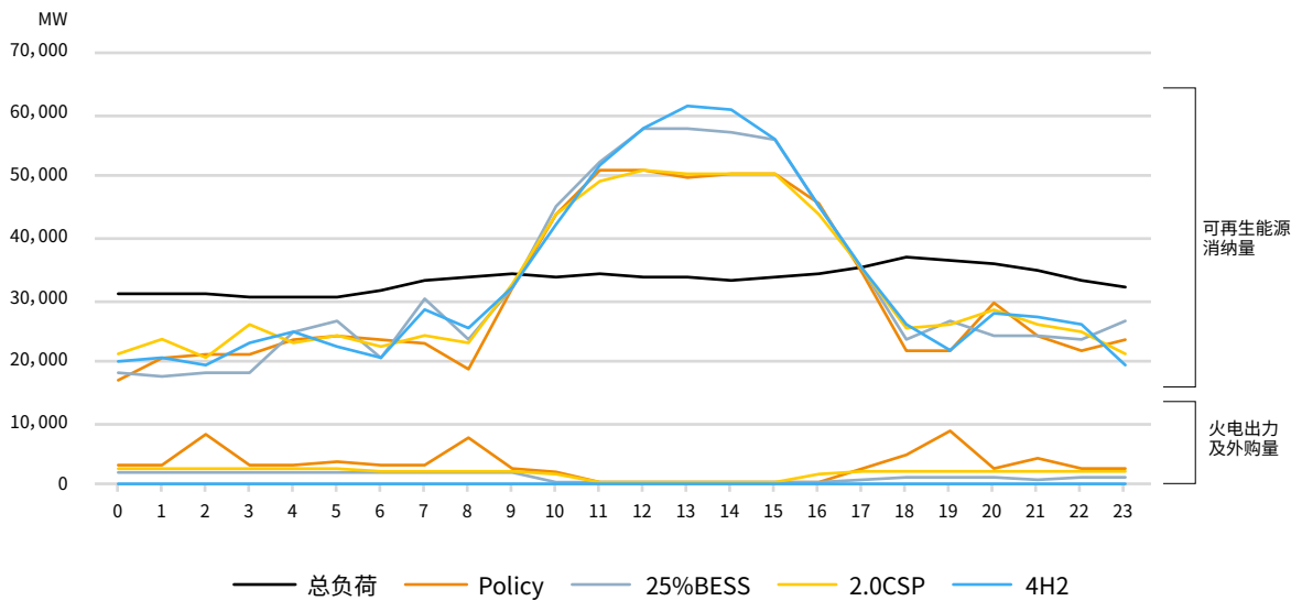
图表 33 枯水期(冬季)典型日可再生能源消纳和火电出力及外购量曲线 xi
