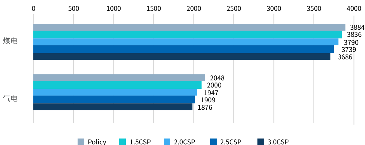
图表 31 不同情景下2021-30年火电年平均利用小时数对比 (剔除利用小时数为0的年份, 不含氢能发电)
