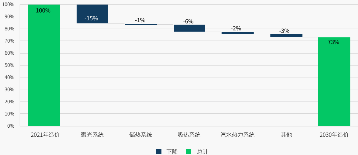
图表 12 塔式光热电站造价成本下降趋势
